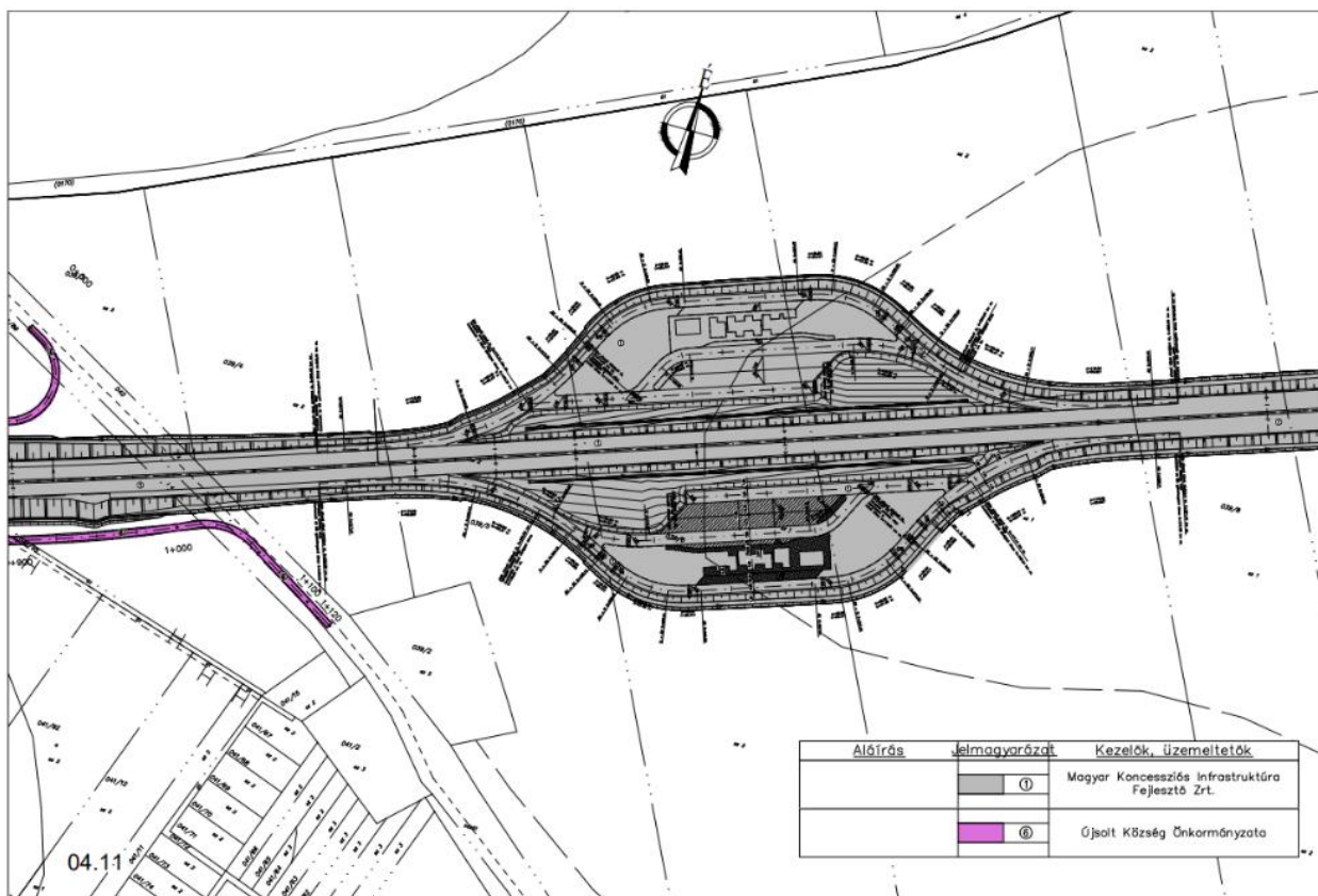
MŰSZAKI RÉSZLETEK FORRÁS: FÖMTERV MÉRNÖKI TERVEZŐ ZRT.
